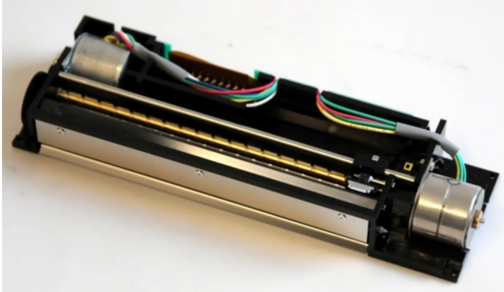
Mechanizm drukujący do drukarek KAFKA, MEFKA.
